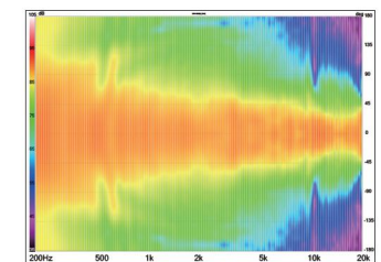
垂直指向性
