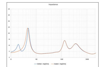
阻抗
